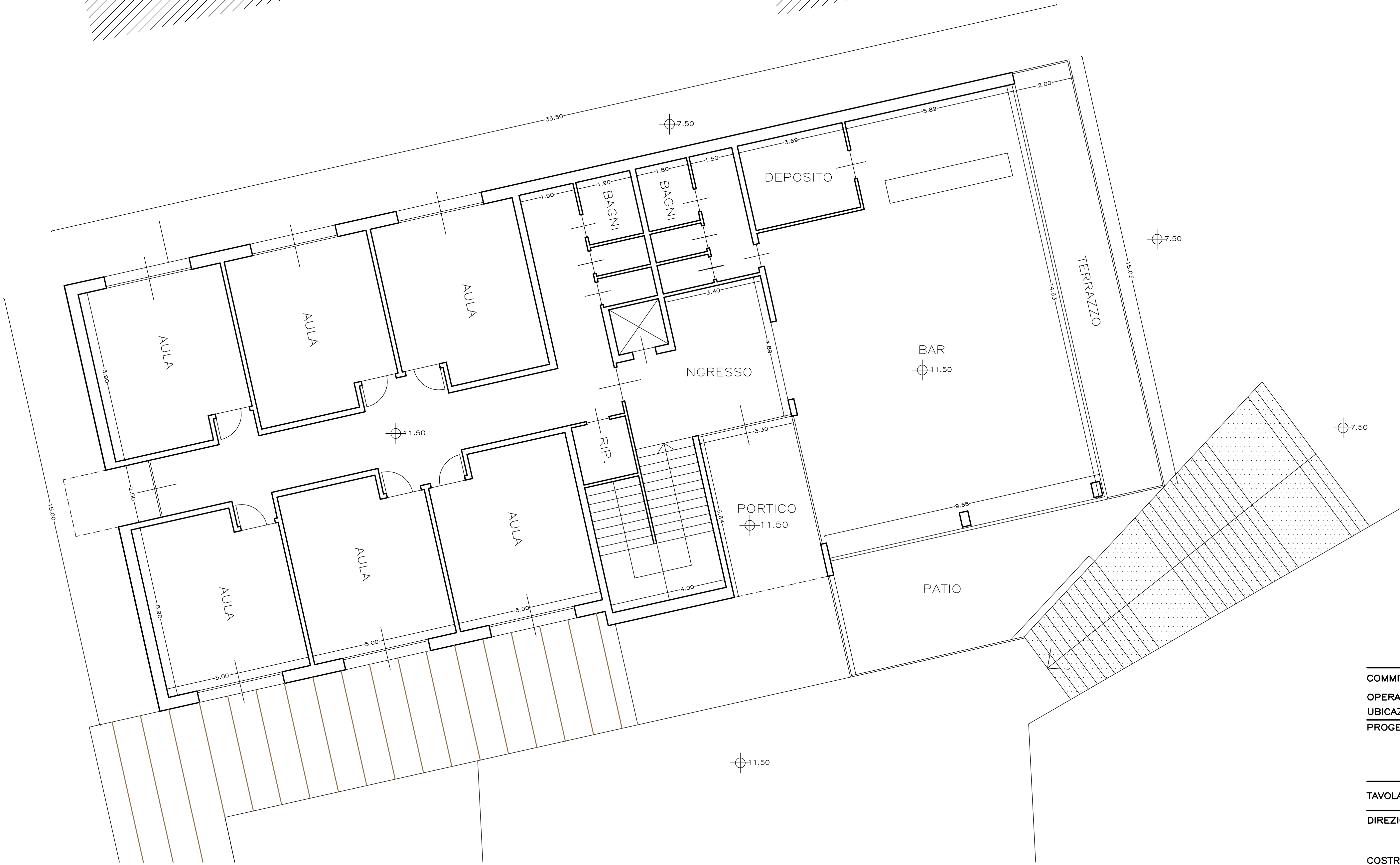
PIANTA PIANO PRIMO — 1:100
